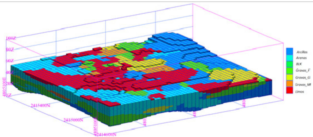
Figura 27. Modelo estratigráfico de un depósito de placer Fuente: autores
